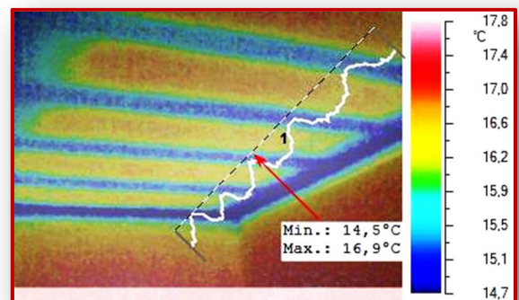
Verifica orditura solai mediante rilievi termografici IR
